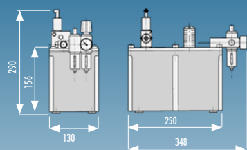
Art.396B blocco base per comando PNEUMATICO
